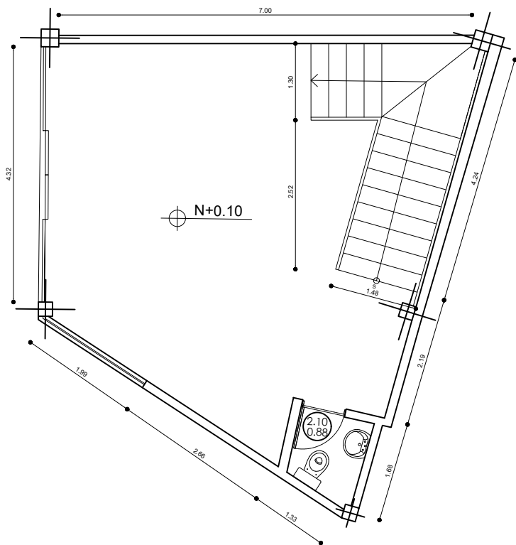
PLANO PRIMER NIVEL Local #7
